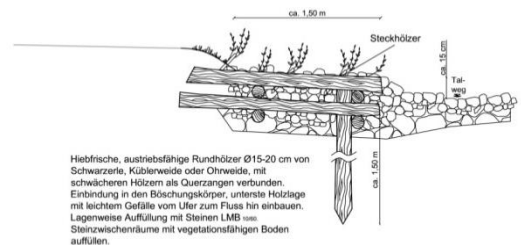
Detail Steinkastenbuhne
