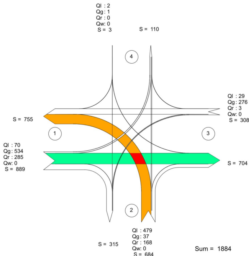
Knotenstromdarstellung mit den am stärksten konkurrierenden Strömen im Kreisverkehr
