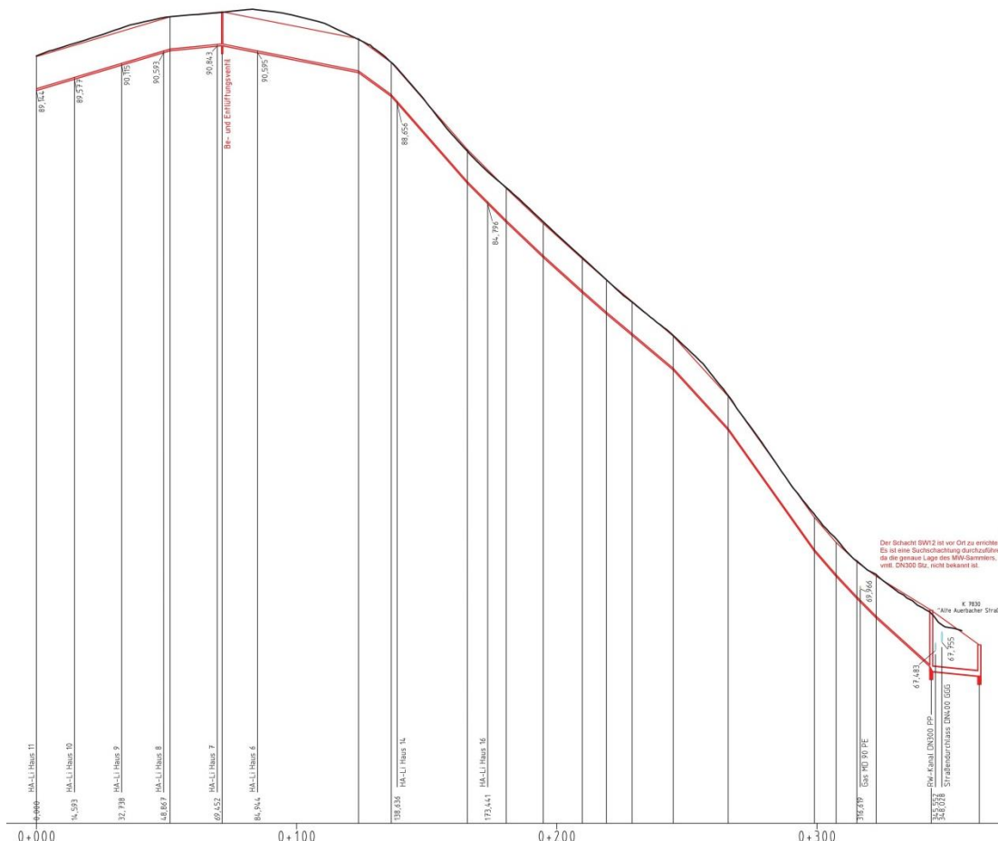
Längsschnitt des Hauptstrangs
