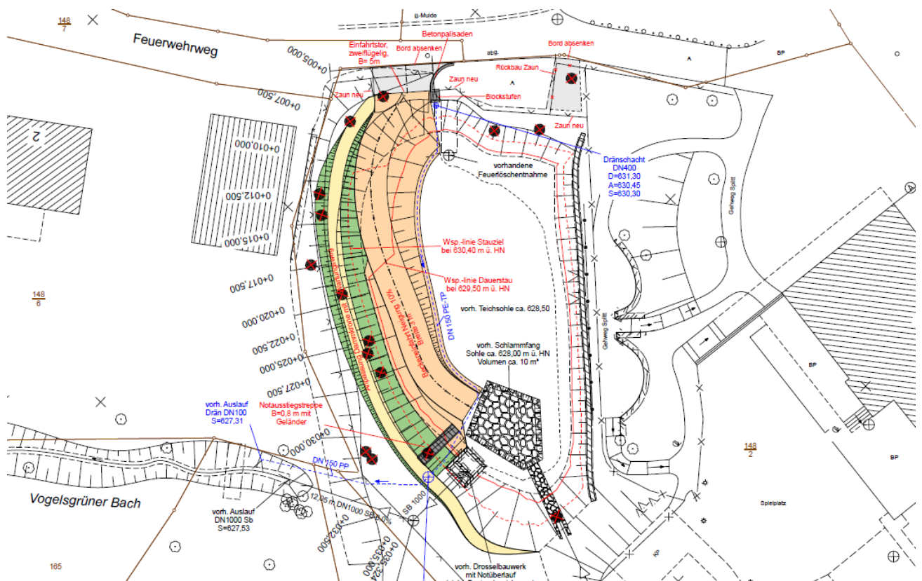
Lageplan mit Beckeneinfahrt und Dammböschung
